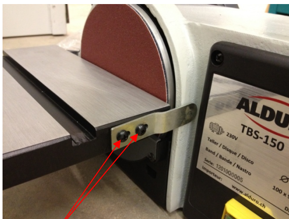
Schrauben/Vis de fixation
